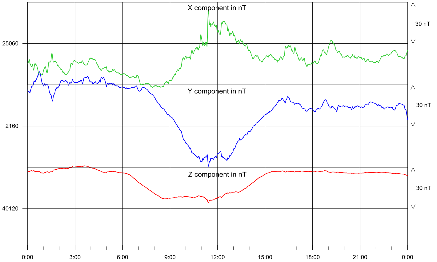
Şekil-1. İznik Manyetik Rasathanesi'nde kaydedilen 2013 Haziran ayı günlük manyetik alan değişimi.
